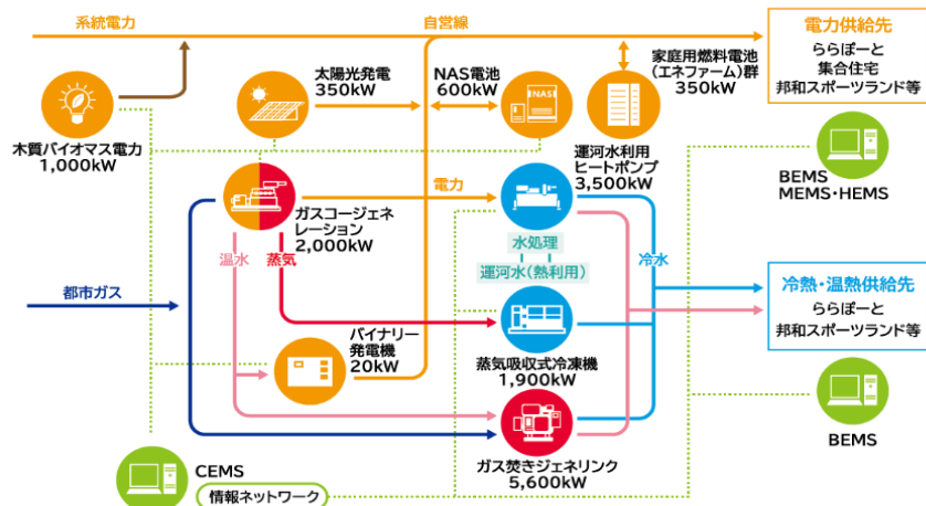
エネルギーシステム構成図
